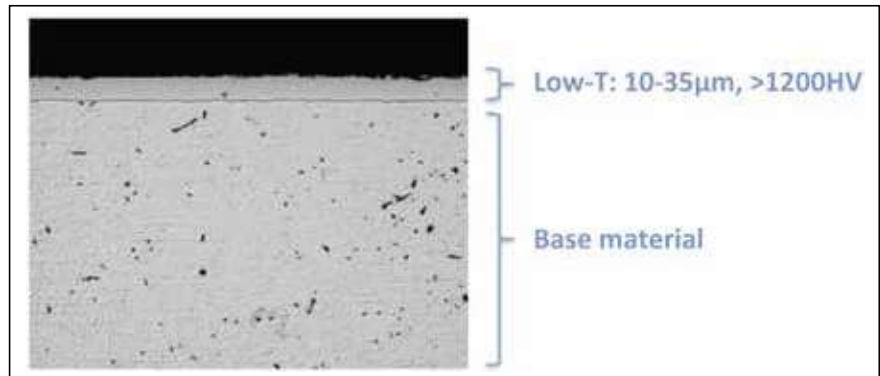
Optisk Micrograf af Expanite-hærdet A 286 (1.4980)-materiale. Lagtykkelsen bliver mellem 10 og 35 µm, og en overfladehårdhed på 1.200-1.500 HV0.05.
