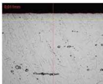
Optisk Micrograf af Expanite-hærdet Inconel 718 viser en homogen lagtykkelse på ca. 10 µm. Hårdhedsmåling viser ca. 1.000 HV0.025.
