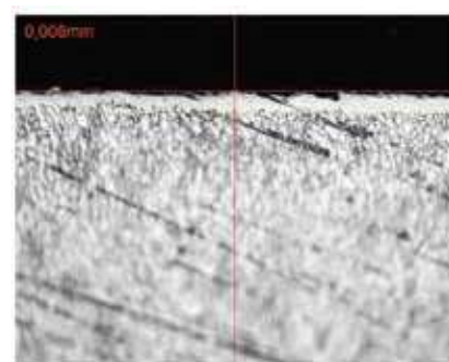
Optisk Micrograf af Expanite hærdet Stellite 1040 viser en hærdet zone på ca. 8 µm. Hårdhedsmålingerne viser ca. 900 HV0.025.
